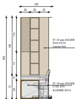
POGLED NA POLICE OD STRANE STOLA
