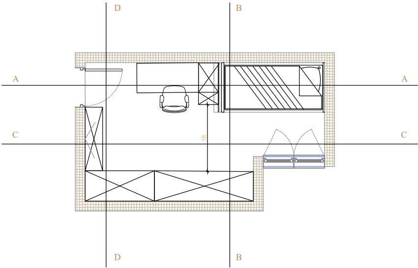
TLOCRT - pogledi i presjeci
