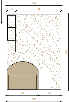
POGLED B
