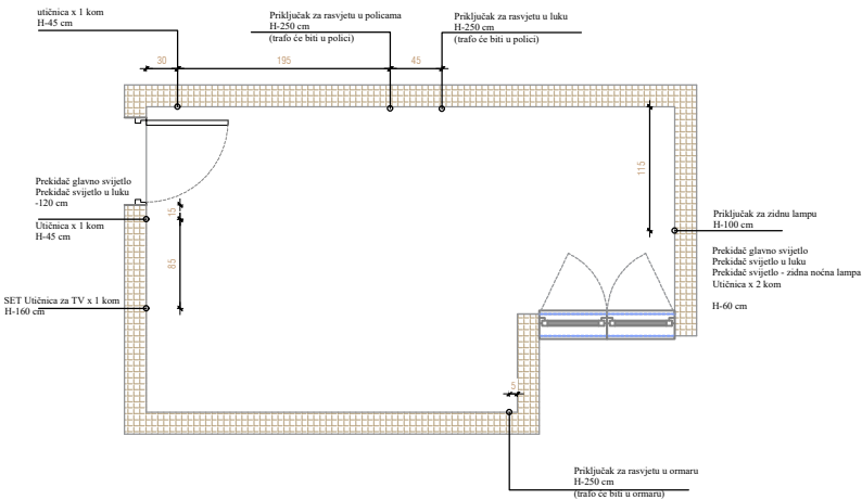
TLOCRT - pozicije elektroinstalacija
