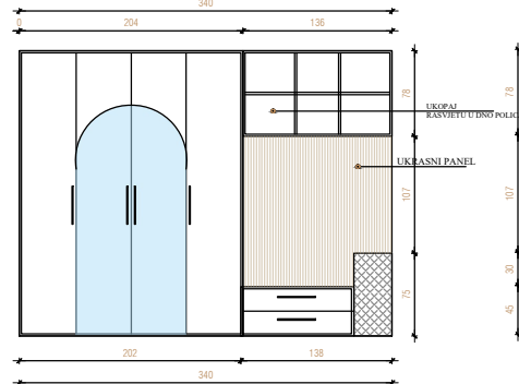
POGLED ORMAR VANI
