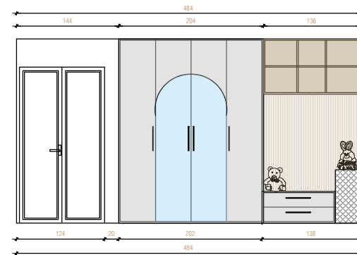
POGLED C
